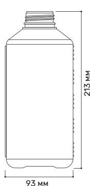
Флакон для локтевого дозатора «Еврофлакон» 1000 мл
