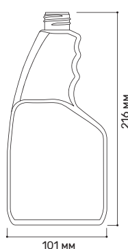
Флакон под триггер «Модерн» 500 мл
