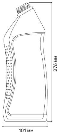
Флакон со скошенным горлом «Элеганс» 750 мл
