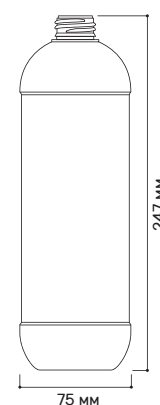
Флакон цилиндрический «Белизна» 900 мл
