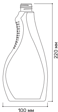
Флакон под триггер «Элеганс» 500 мл
