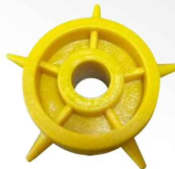
Катушка высевальная сеялки Тетро 499655/491615
