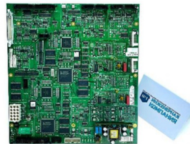
ЭЛЕКТРОННЫЕ ПЛАТЫ
