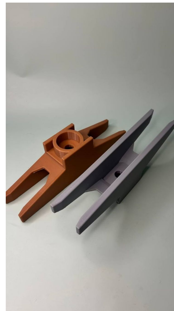
Направляющие на конвейере шоколадных конфет
